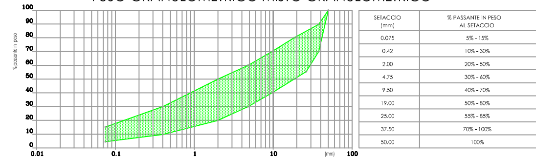
FUSO GRANULOMETRICO MISTO GRANULOMETRICO
